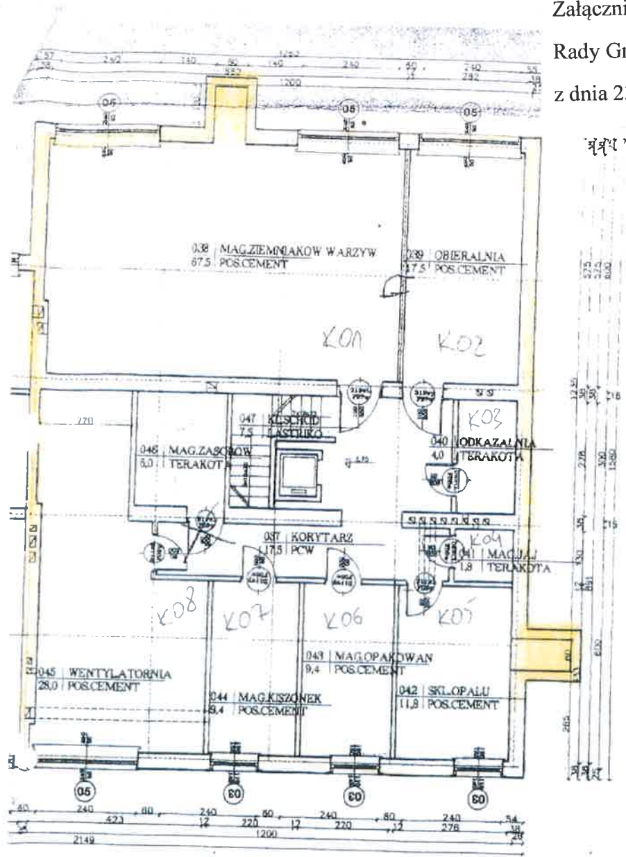
RZUT PIWNIC 1:100
